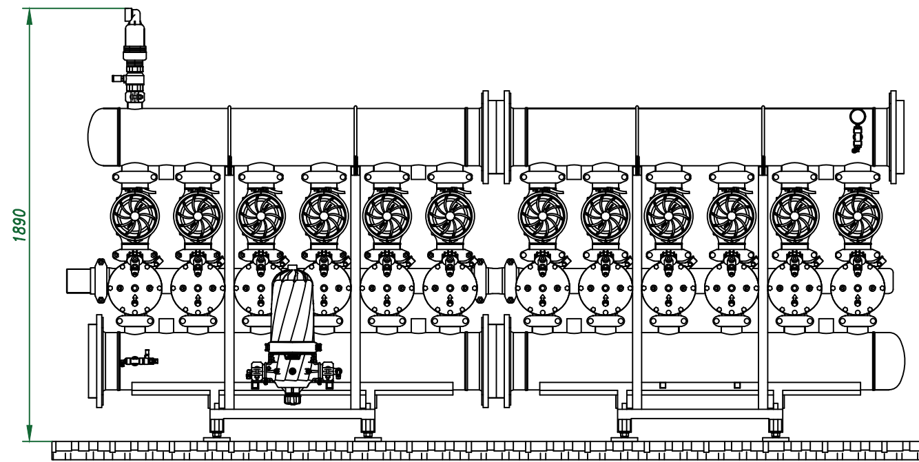
Вид спереди
